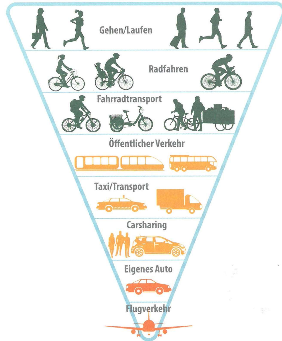
Umgekehrte Verkehrspyramide
